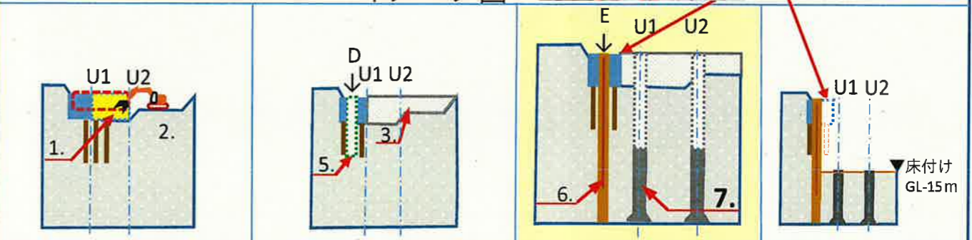
③エキスパンションジョイントの増
