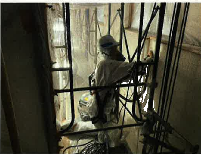
【外壁仕上塗材石綿除去作業状況】
