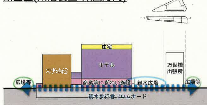
断面図(川沿街区・東西方向)
