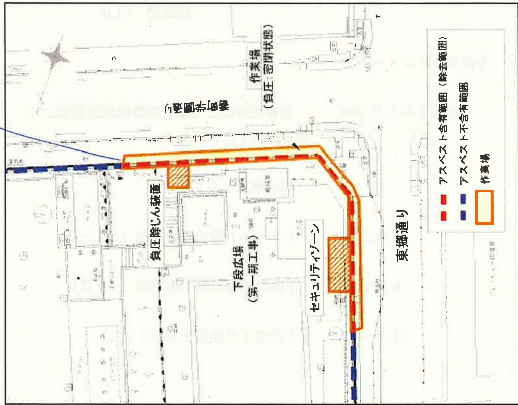
■アスベスト含有範囲・設備配置
